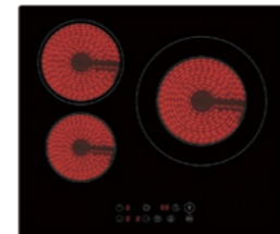
에넥스 3구 하이라이트 TAE-T301 - 화구 : 3구 하이라이트 - 치수 : W580 × D510 - 타공 : W560 × D480 - 매입깊이 : 45mm
