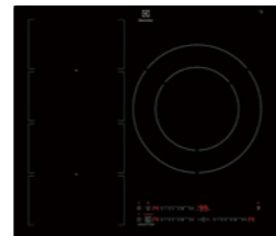
일렉트로룩스 인덕션 CIV65344 - 화구 : 3구 인덕션(와이드존) - 치수 : W590 × D520 - 타공 : W560 × D490 - 매입깊이 : 45mm - 공급처 : 일렉트로룩스(독일)
