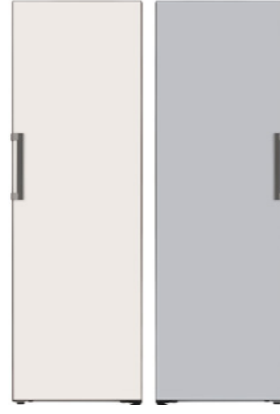
LG 오브제 컨버터블 냉장/냉동고 (냉장 6종/냉동 6종 - 색상동일) - 용량 : 냉장고384l / 냉동고321l - 치수 : W595 × D670 × H1860mm - 전용장 : CAR-62CM ※ PRM / ENEX CAD 참고(컬러)
